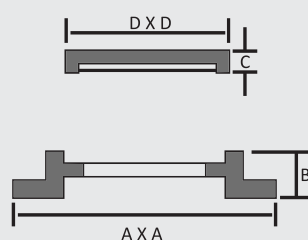
Grelha alto tráfego padrão portos e aeroportos Resistência d-400 E-600 F-900
