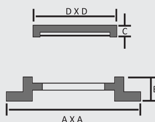
Tampa Articulada Telefone R - 2 TPFO
