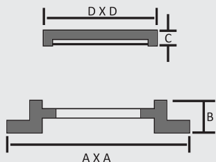
Tampa Padrão Telefonica R - 2
