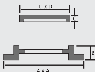
Grelha GR-135 Articulada Padrão Aeroporto
