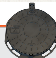
Tampão TDA - 600 Padrão Aeroporto Com anel anti-ruído Resistência E - 600 F - 900
