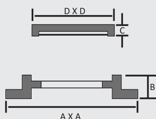
Tampa Articulada Telefone R - 2
