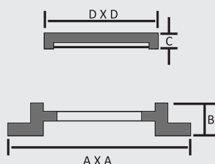
Grelha GR-135 Articulada
